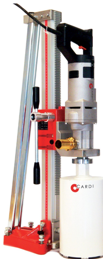
CARDI 183 - Motor T2000 Me-14 + L180 stander 2000W - Kapacitet Ø32 til Ø202 Integreret udsugningssystem.
